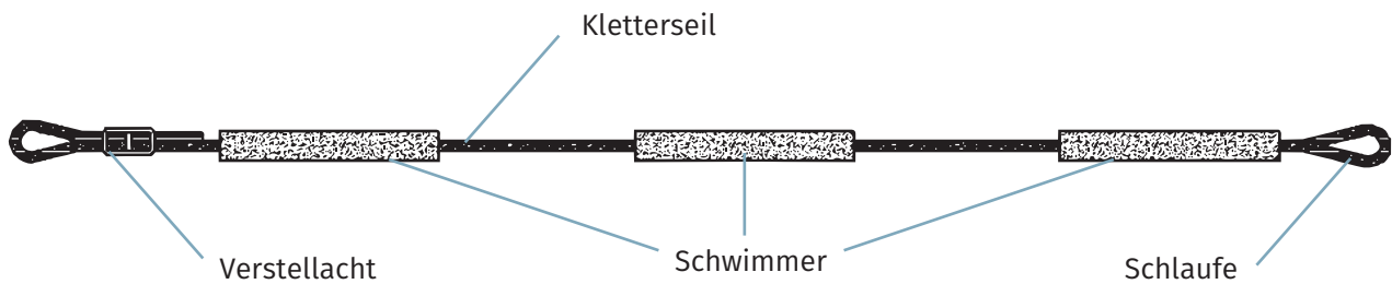
Abb. 1: Aufbau der Kletterleine
